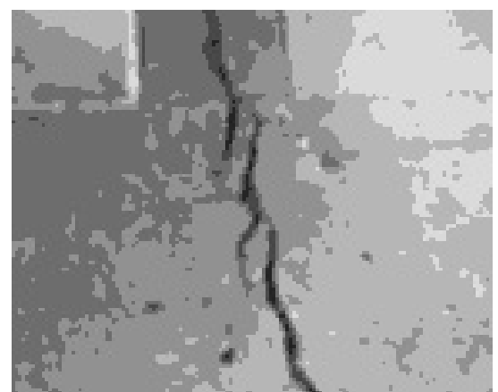
写真 - 4 階調化した画像（丸印拡大）
