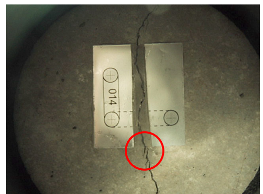
写真 - 3 ひびわれの撮影画像
